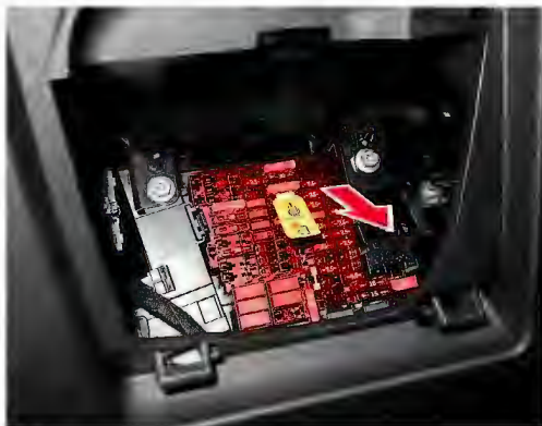
Rettungstrennstelle Sicherungsträger
