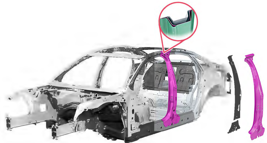
B-Säule mit mehrschaligem Aufbau
