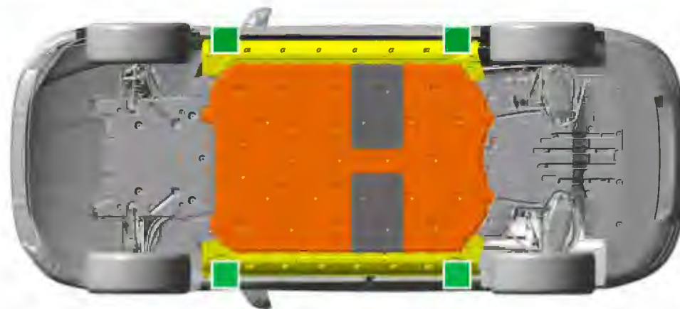
Geeignete Hebepunkte am Beispiel Audi e-tron GT
