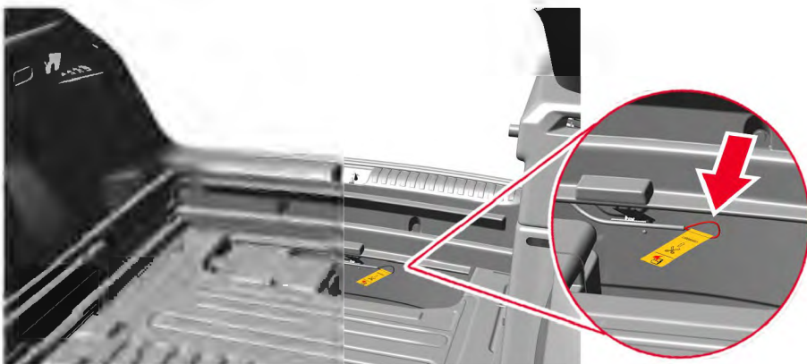
Trennstelle im Gepäckraum Q4 e-tron unter dem Kofferraumboden am Heckabschluss. Das gelbe Fähnchen kennzeichnet die Trennstelle.
