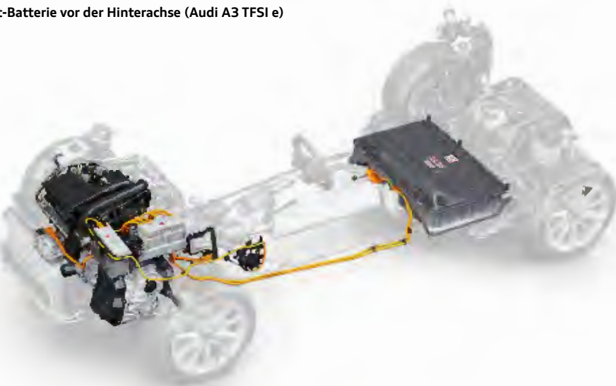
Hochvolt-Batterie vor der Hinterachse (Audi A3 TFSI e)
