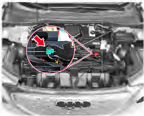
Trennstelle im Motorraum Audi Q4 e-tron
