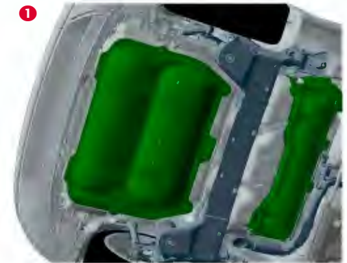
1 Tankabdeckungen am Unterboden entfernen. Die Tankabdeckungen sind in dieser Abbildung grün gekennzeichnet.
