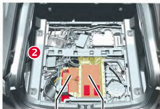
12-Volt-Batterie 48-Volt-Batterie
